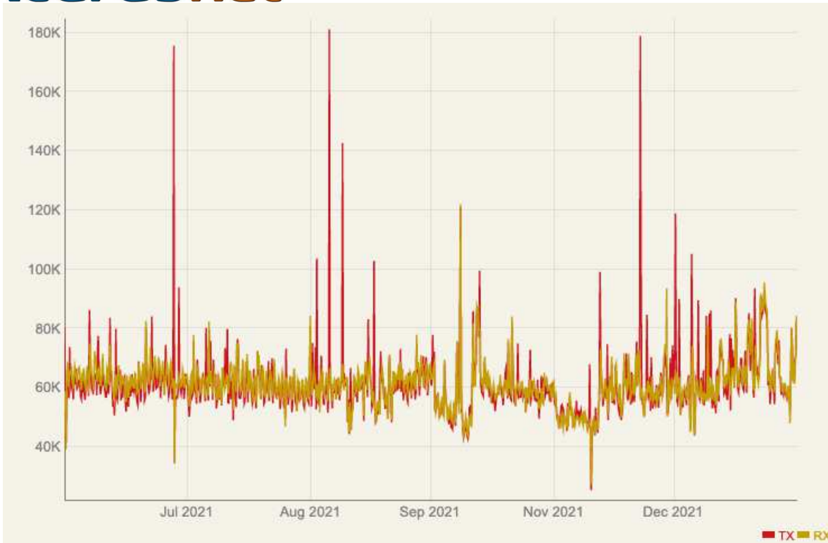
Fig. 1 – Traffico trasmesso/ricevuto rete Enas 01/07/2021 – 31/12/2021
